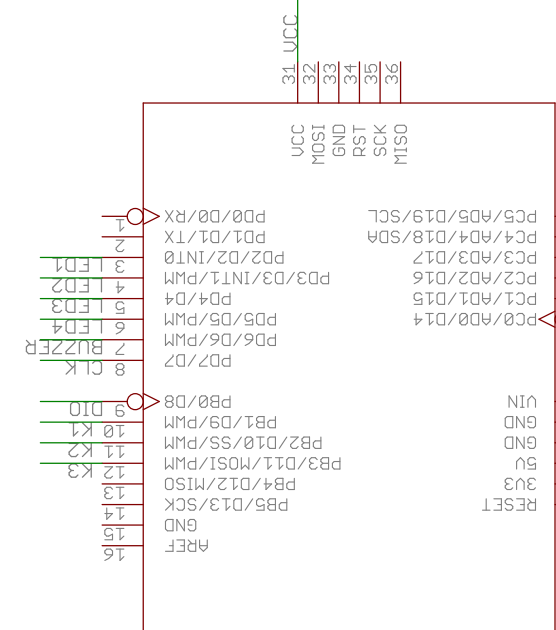
ARDUINO SHIELD
